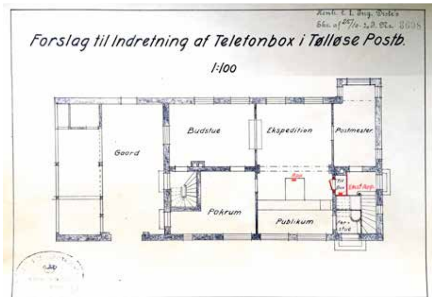
Grundplan over posthuset i Tølløse. Enigma/Postmuseet.
