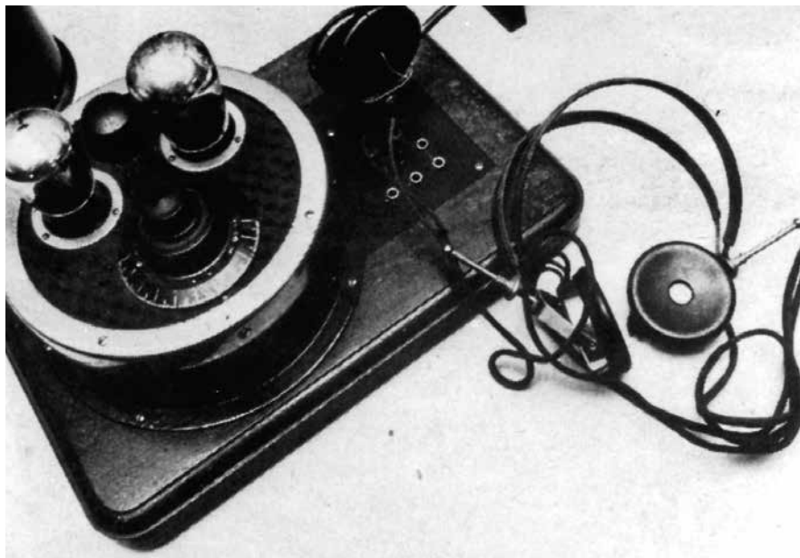
Batteridrevet radiomodtager fra Ugerløse Maskinfabrik, bygget ca. 1925.
